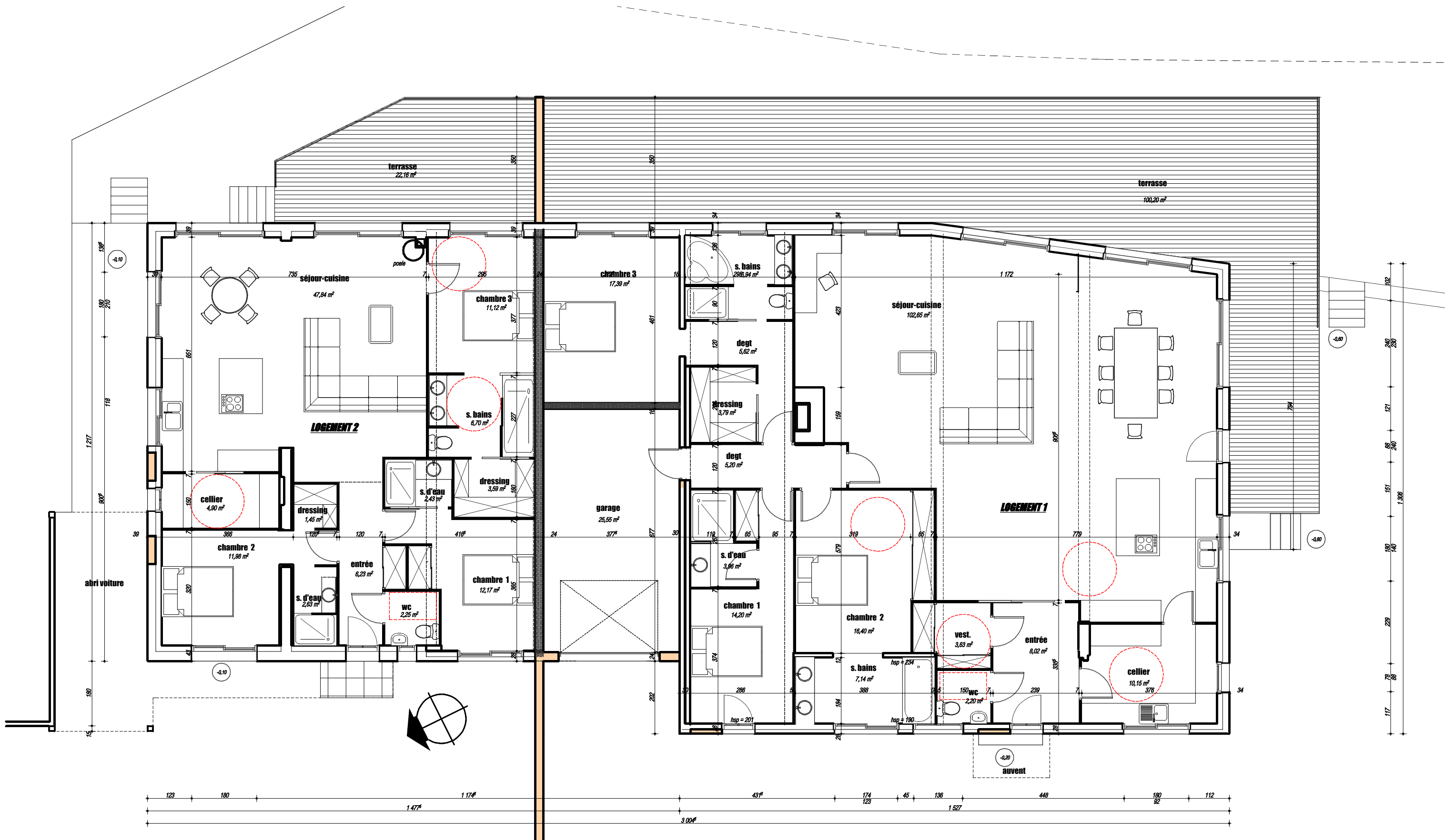
Plan rez-de-chaussée projeté Echelle 1/75 e
